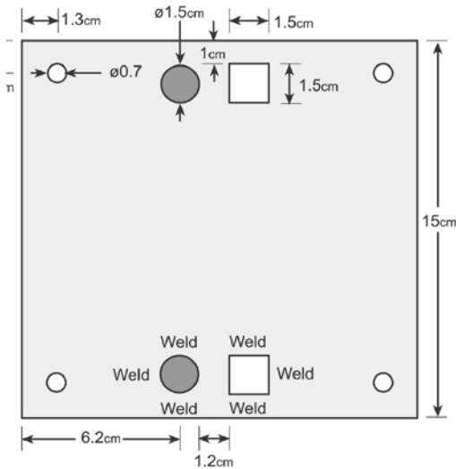
Base del Blanco (Vista de Planta)
